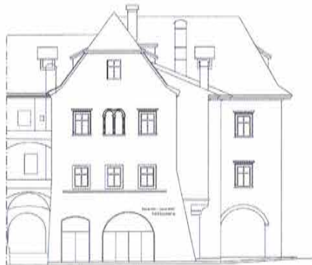
Ansicht Süd Prospetto sud
